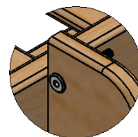
DÉTAIL A ECHELLE 1 : 5
